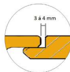
Tekening 10 Volgende expansieruimte aanhouden tussen delen.
